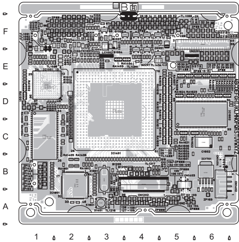
<02> DIGITAL LPB10236-001D -FOIL SIDE-
